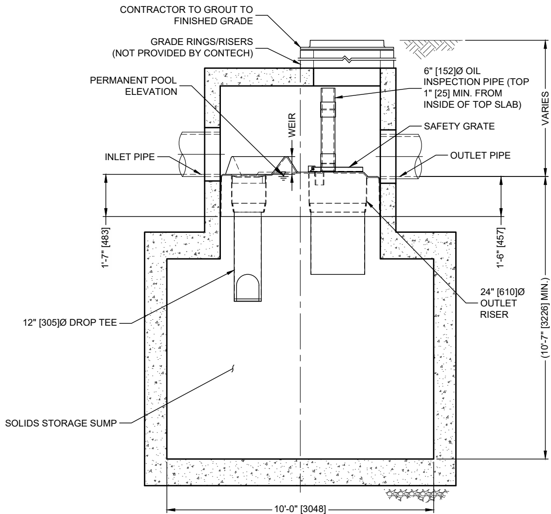
SECTION A-A
