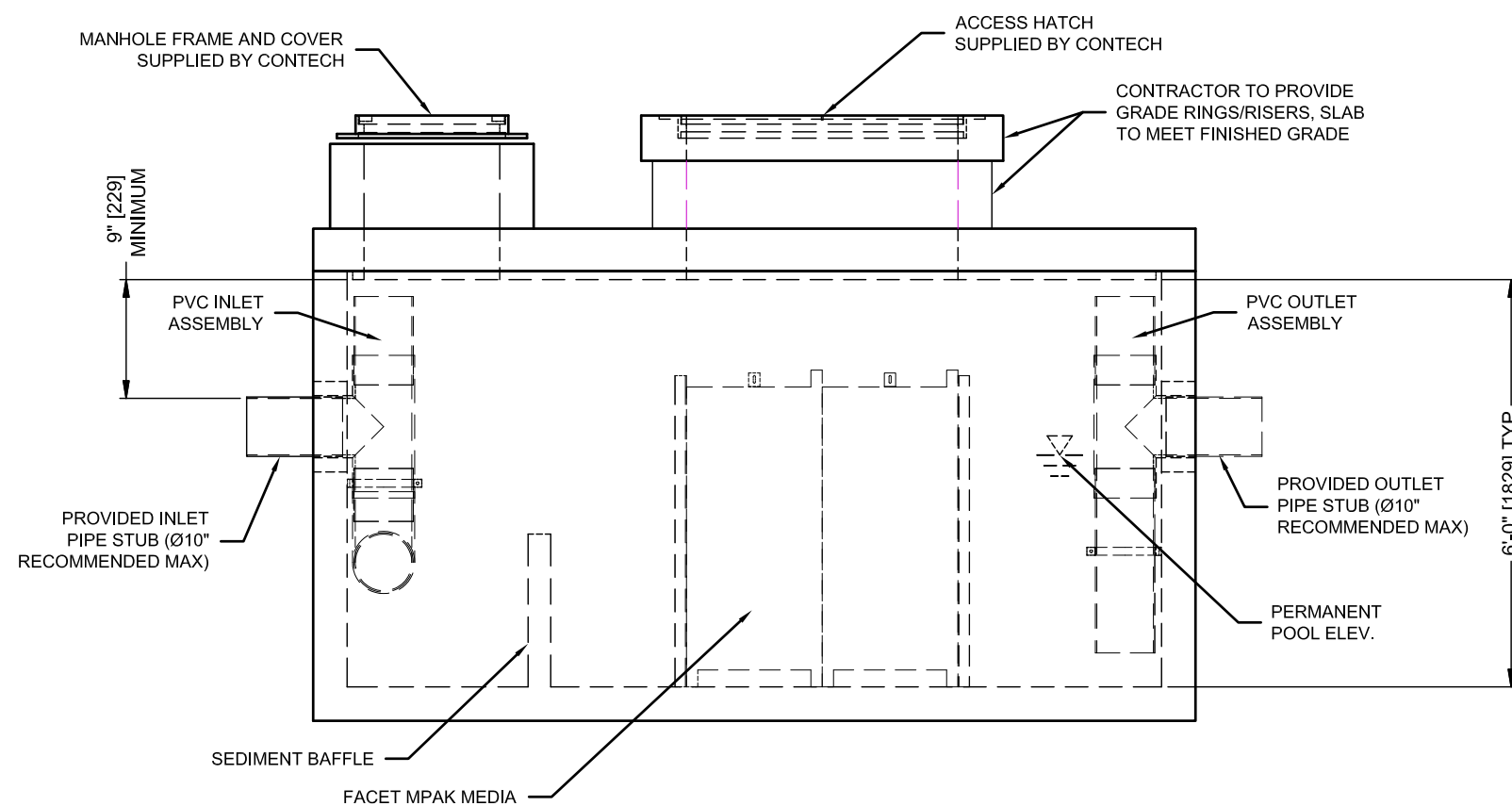
ELEVATION VIEW VortClarex®
