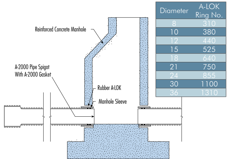
12"-36" manhole gasket
