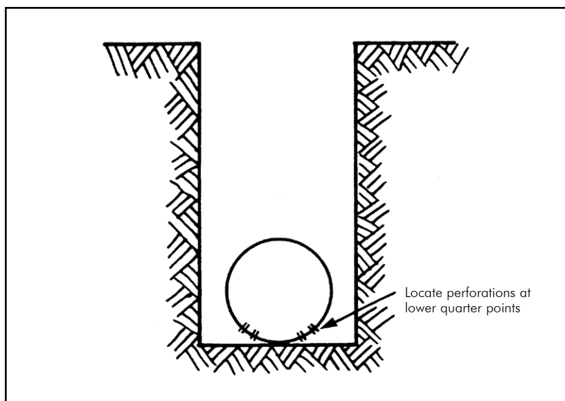
Figura 29. Colocación correcta de los subdrenes de acero perforado.
