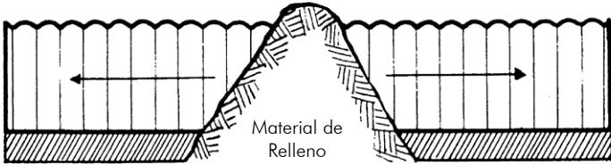
VISTA LATERAL - Sin Cabeceras
