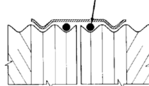
Semi-Corrugada (Abrazadera)
